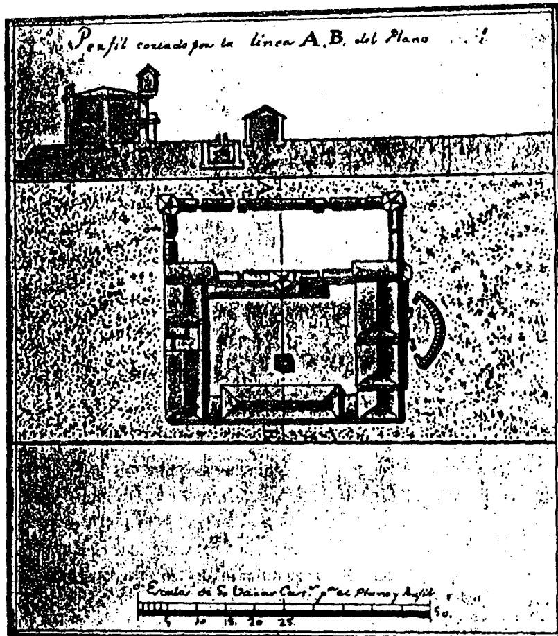
La casa-fuerte de Santa Cruz del Romeral después de la reforma de 1770. Plano de Miguel Hermosilla.
